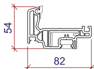
Flügel-Profil A343 - Grösse 54 mm Profil de vantail A343 - grandeur 54 mm
