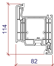
Sockel-Aufbauprofil Z92 Profil de socle Z92
