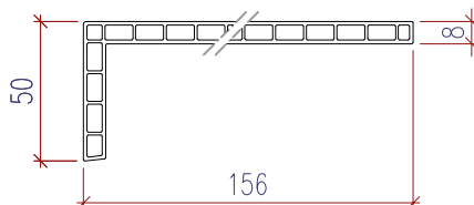
Art. 111.032 Winkel-Profil 156x50 mm Profil d'angle 156x50 mm
