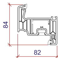
Flügel-Profil A347 - Grösse 84 mm Profil de vantail A347 - grandeur 84 mm
