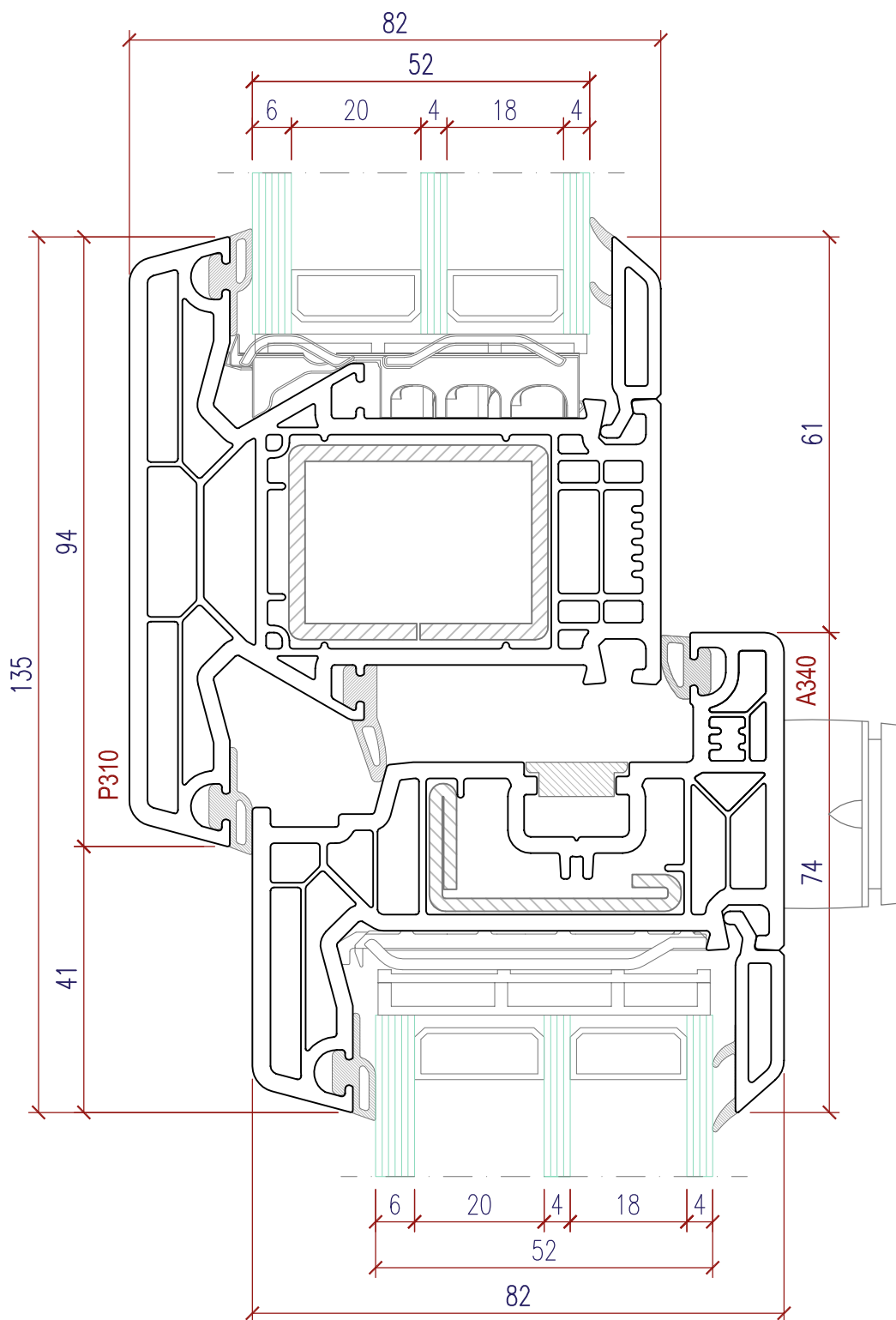
Profilkombination - Flügel / Fixverglasung : P310 - A340 Combinaison - vantail / verre fixe
