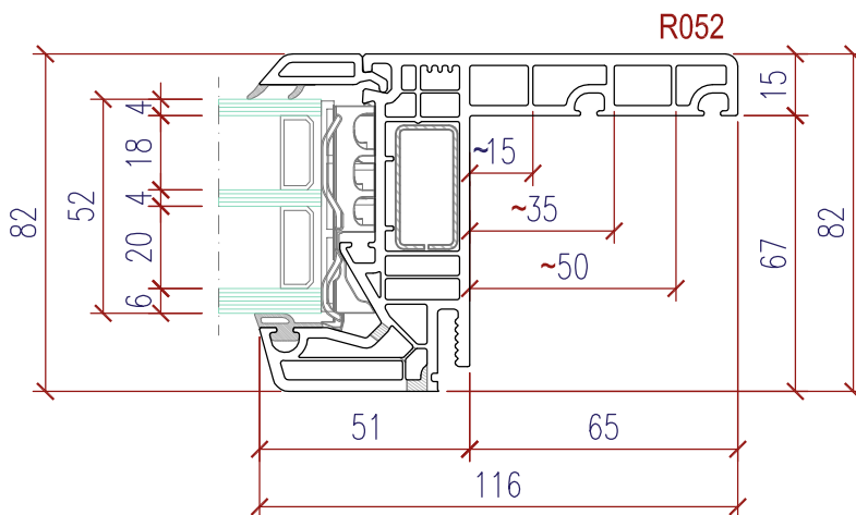
Fix im Rahmen verglast : R052 Fixe dans le cadre
