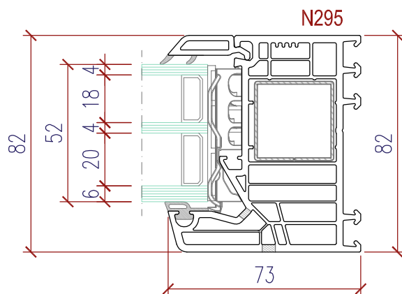
Fix im Rahmen verglast : N295 Fixe dans le cadre
