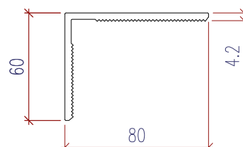
Art. 111.033 Profil/ Profil 6x7.7 mm
