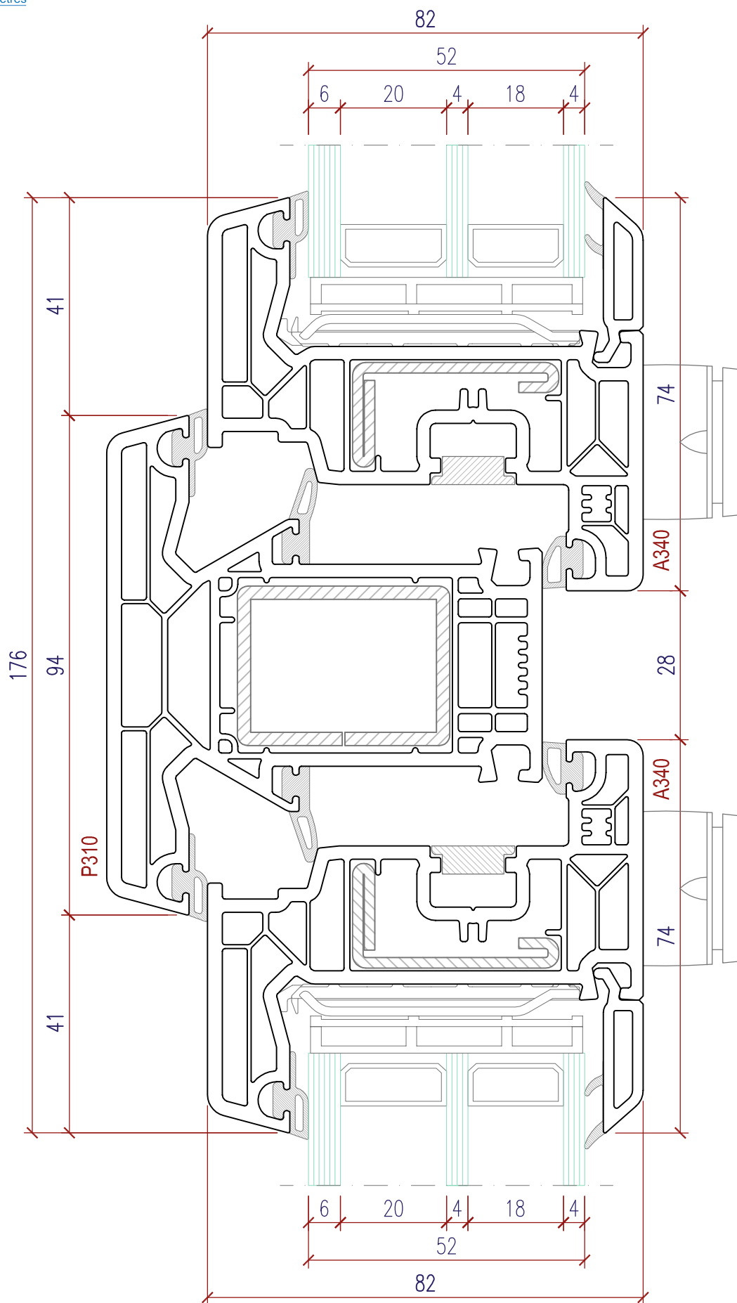
Mittelpartie mit Pfosten : P310 - A340 Partie centrale avec/montant
