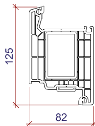
Profil für Fenster-Türe A381 Grösse 125mm für grosse Türen nach AUSSEN öffnend Profil pour porte fenêtre A381 grandeur 125mm pour grandes portes ouv. à l'extérieur
