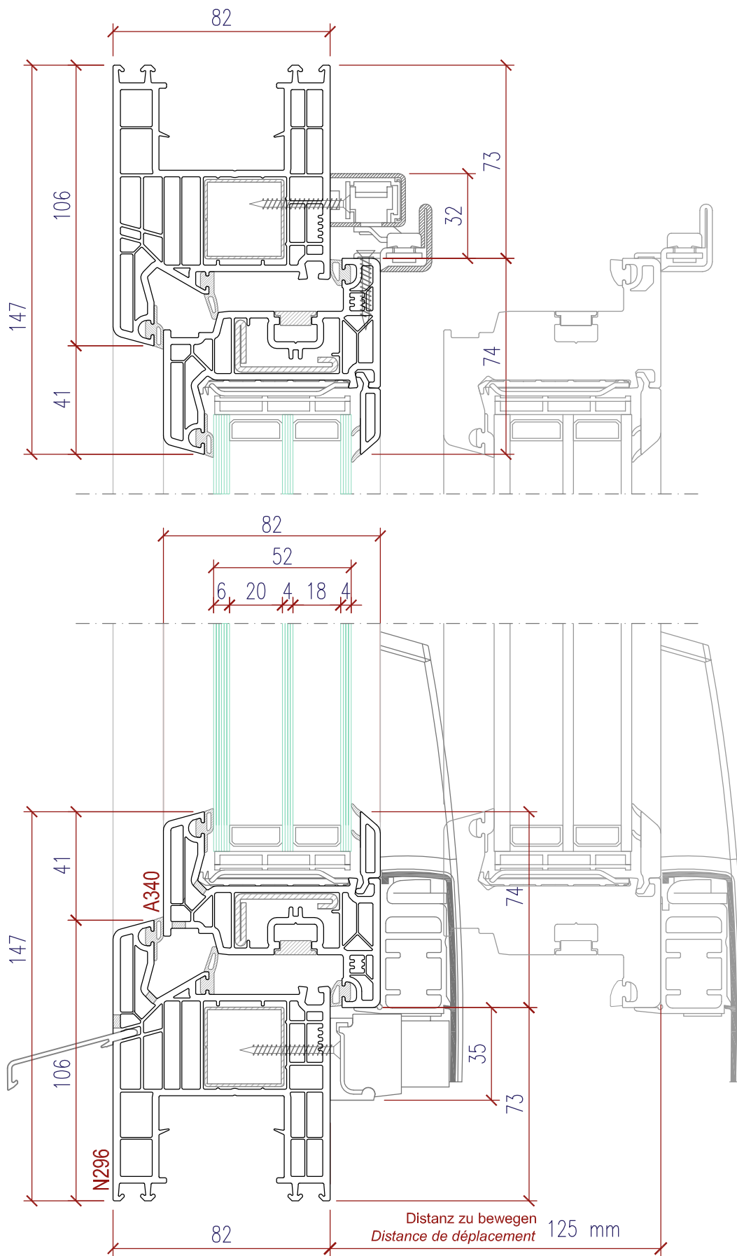
Paralell-Schiebe-Türe PSK Fenêtre translation PSK
