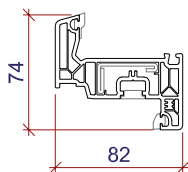
Flügel-Profil A343 - Grösse 54 mm Profil de vantail A343 - grandeur 54 mm
