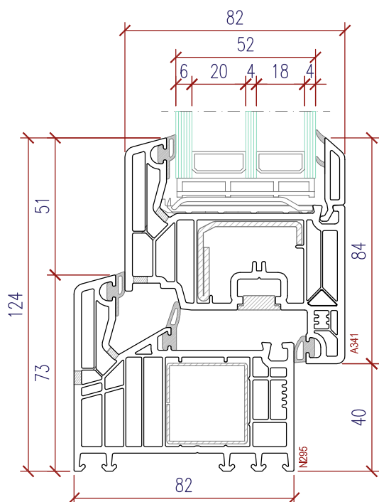
Profilkombination - Rahmen/FI ügel : N295 - A341 Combinaison - cadre/vantail
