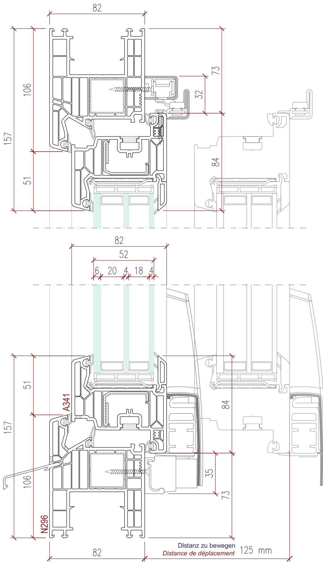
Paralell-Schiebe-Türe PSK Fenêtre translation PSK
