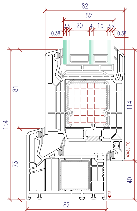
Profilkombination - Rahmen/FI ügel : N295 - A345/TS Combinaison - cadre/vantail
