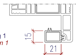
Art. 109.531 Profil/ Profil 21x15 mm
