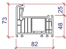
Profilkombination - Rahmen / Flügel N293 Combinaison - cadre / vantail N293
