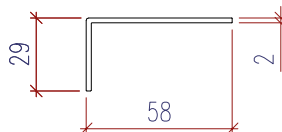
Art. 109.001 Winkel-Profil 60x40 mm Profil d'angle 60x40 mm
