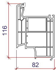
Sockel-Aufbauprofil Z92 Profil de socle Z92
