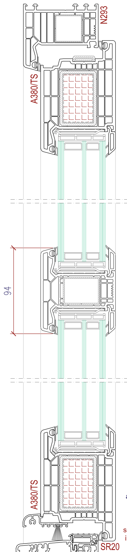
Schnitt A Coupe A
