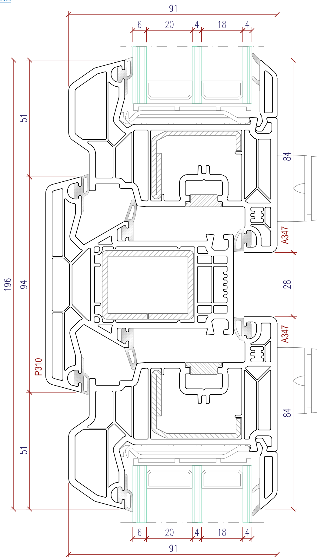
Mittelpartie mit Pfosten : P310 - A347 Partie centrale avec/montant
