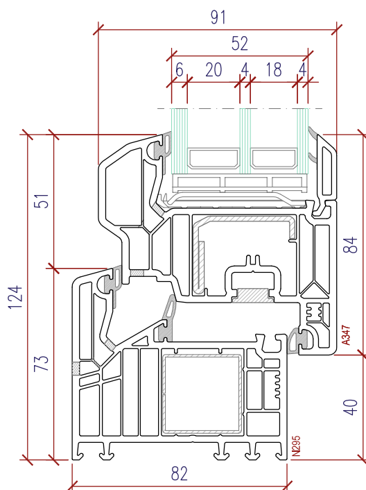
Profilkombination - Rahmen/FI ügel : N295 - A347 Combinaison - cadre/vantail
