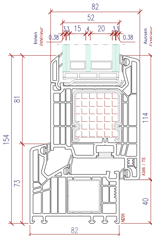
Profilkombination - Rahmen/FI ügel : N295 - A346/TS Combinaison - cadre/vantail
