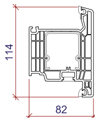
Profil für Fenster-Türe A346 Grösse 114mm für grosse Türen nach AUSSEN öffnend Profil pour porte fenêtre A346 grandeur 114mm pour grandes portes ouv. à l'extérieur
