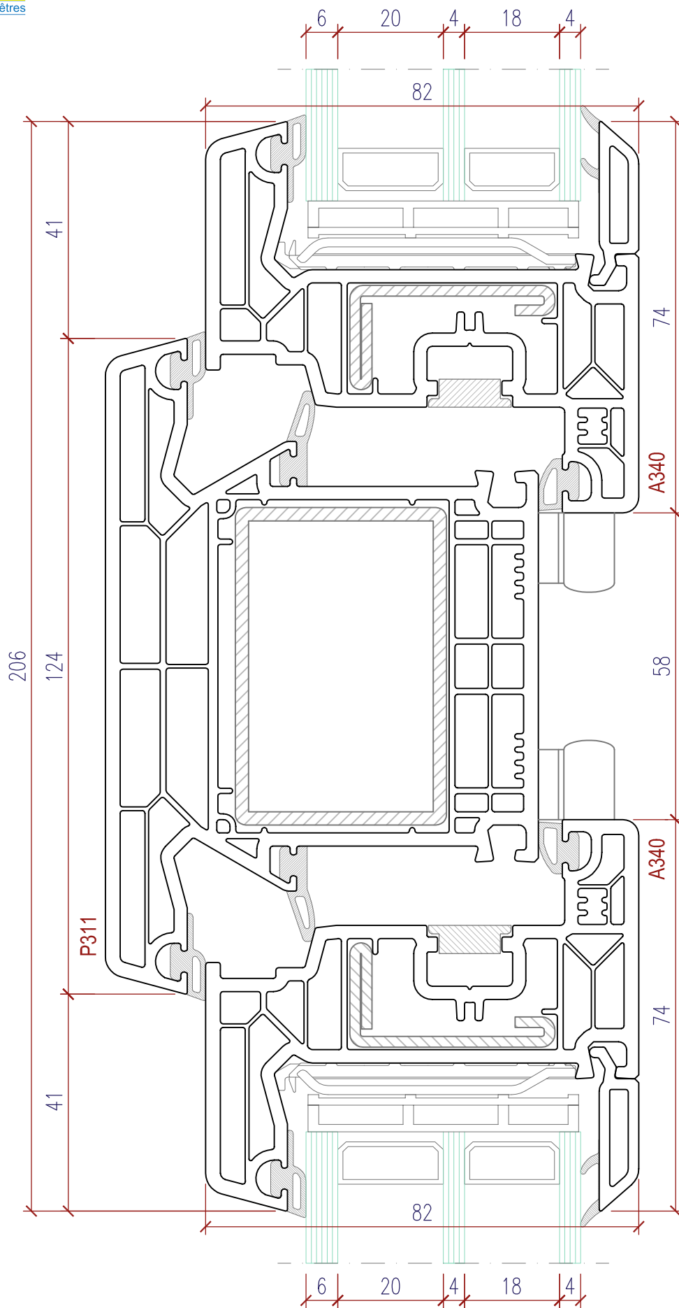
Mittelpartie mit Pfosten : P311 - A340 Partie centrale avec/montant
