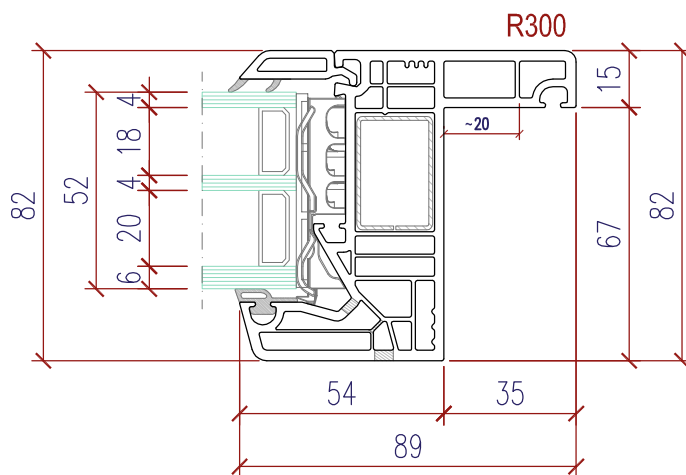
Fix im Rahmen verglast : R252 Fixe dans le cadre
