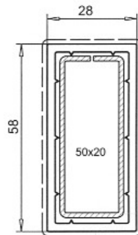
Vorsatzzarge 28x58mm Art.-Nr. 109.082 Verstärkung Art.-Nr.113.047 I_x=1,41\text{cm}^4 , I_y=6,21\text{cm}^4 Verstärkung Art.-Nr.113.047.2 I_x=1,76\text{cm}^4 , I_y=7,86\text{cm}^4 Verstärkung Art.-Nr.113.047.3 I_x=2,33\text{cm}^4 , I_y=10,90\text{cm}^4
