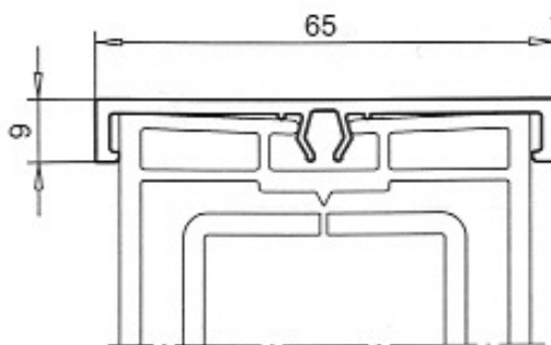
Abdeckprofil Art.-Nr. 109.292 für Zarge Art.-Nr.114.003
