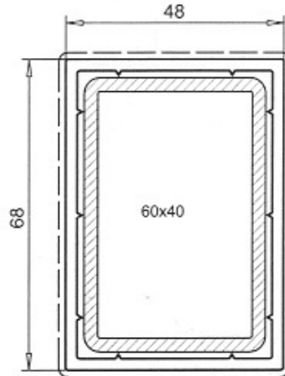
Vorsatzzarge 48x68mm Art.-Nr. 109.081 Verstärkung Art.-Nr.113.011.2 I_x=10,23\text{cm}^4 , I_y=19,31\text{cm}^4 Verstärkung Art.-Nr.113.011.3 I_x=14,32\text{cm}^4 , I_y=27,39\text{cm}^4
