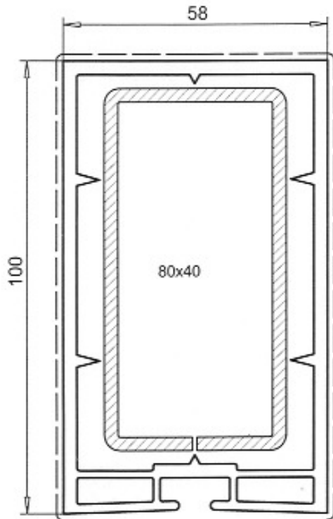
Vorsatzzarge 58x100mm Art.-Nr. 114.003 Verstärkung Art.-Nr.113.015.3 I_x=18,50\text{cm}^4 , I_y=55,50\text{cm}^4
